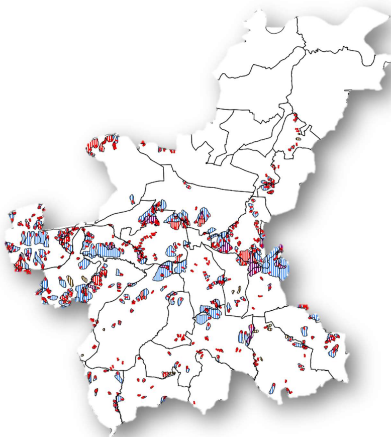
Rysunek 18. Rozmieszczenie osuwisk różnego typu na terenie gminy Wieliczka.
